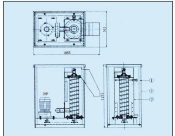
粉碎机502DP/702DP
